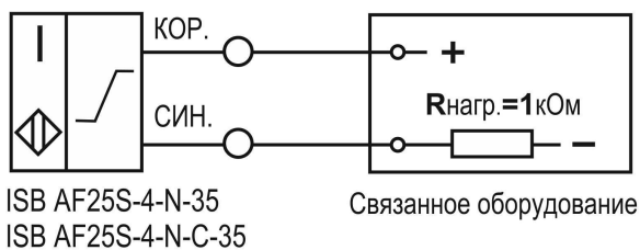
Схема подключения к оборудованию
