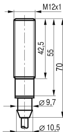
Габаритный чертеж
